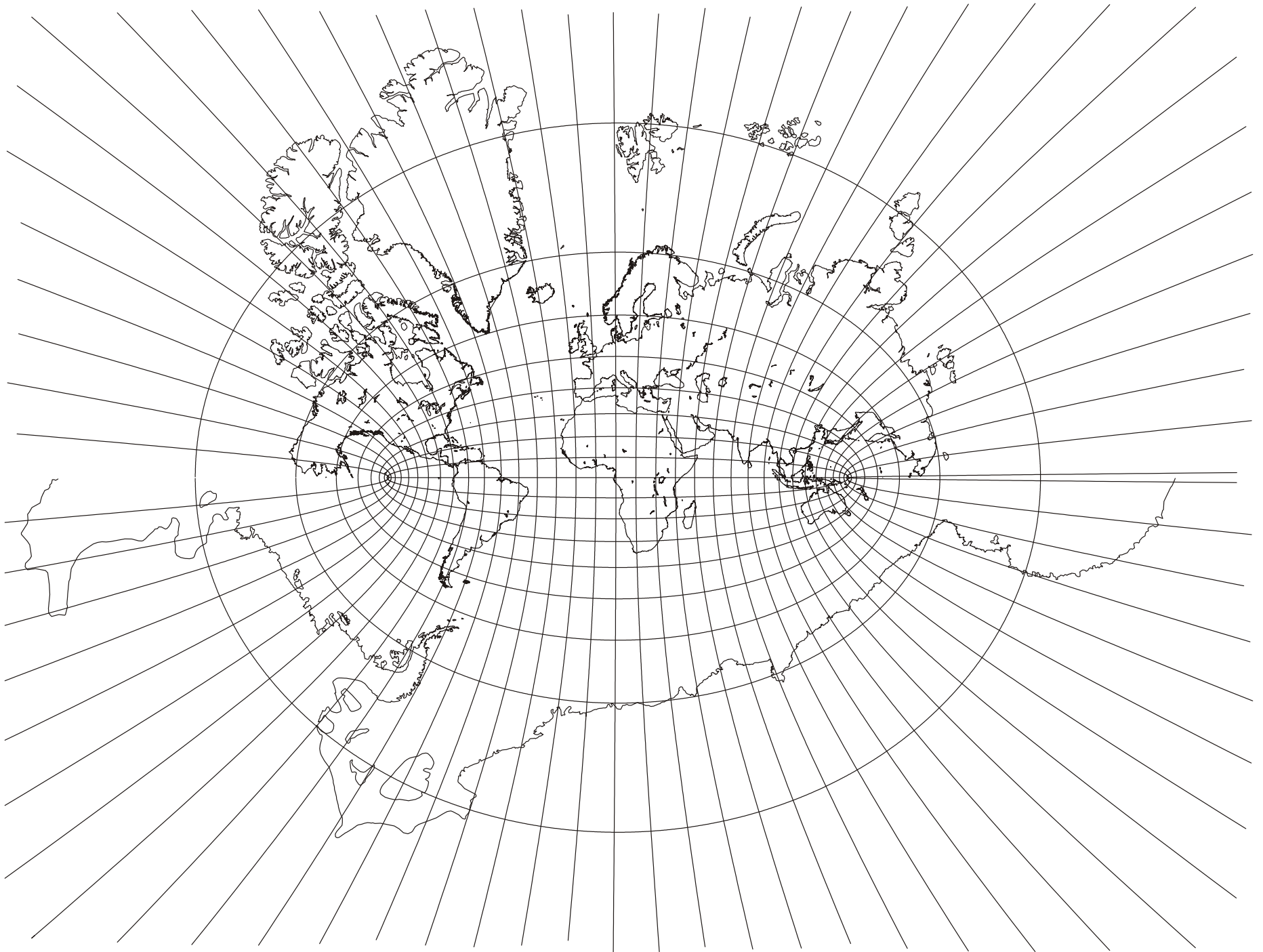
Littrow-Lagrange projection; Retroazimuthal; Conformal;
